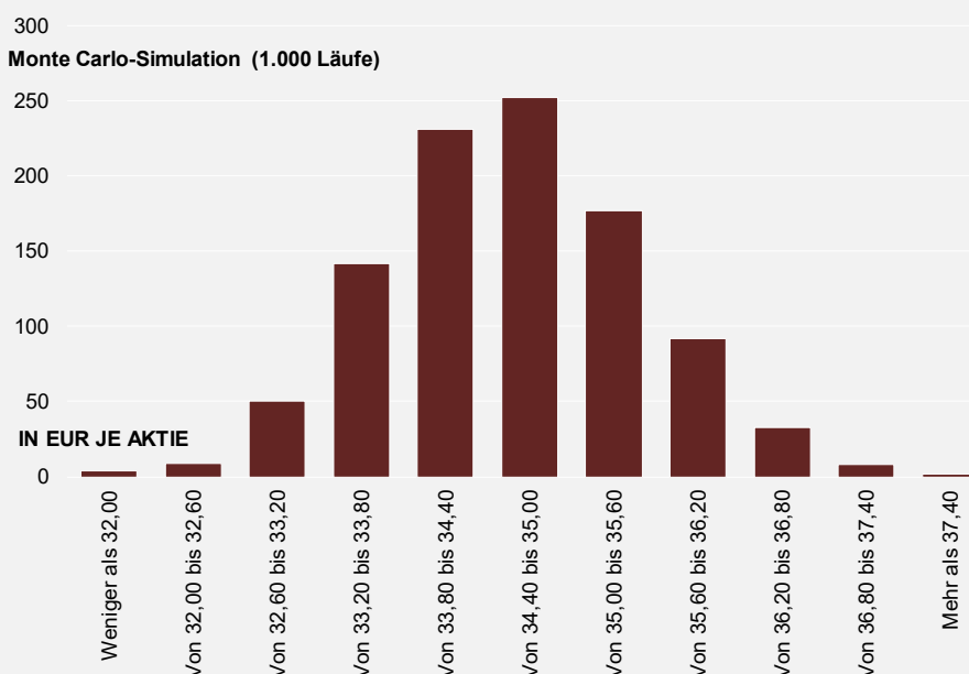
ABBILDUNG 1: MONTE CARLO-SIMULATION (1.000 LÄUFE)
