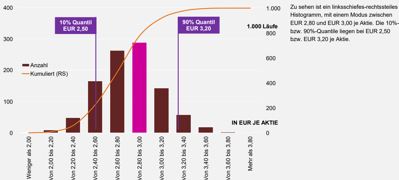
ABBILDUNG 1: MONTE CARLO-SIMULATION
